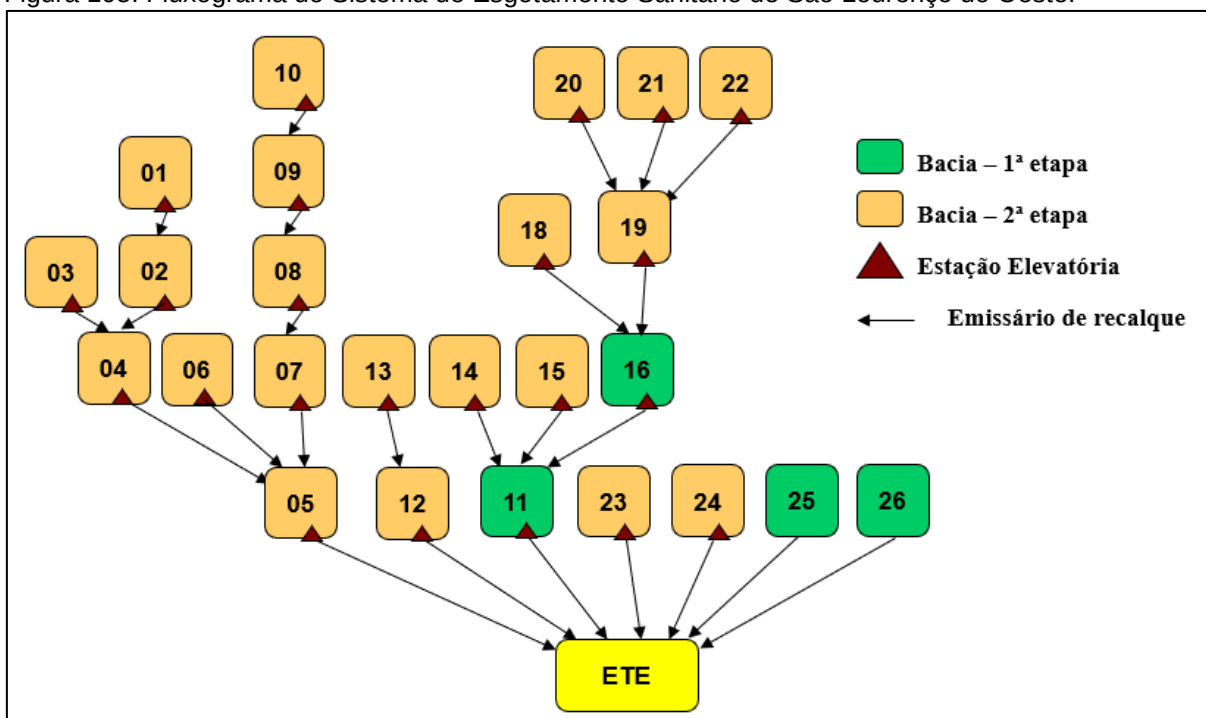
Figura 105: Fluxograma do Sistema de Esgotamento Sanitário de São Lourenço do Oeste.
