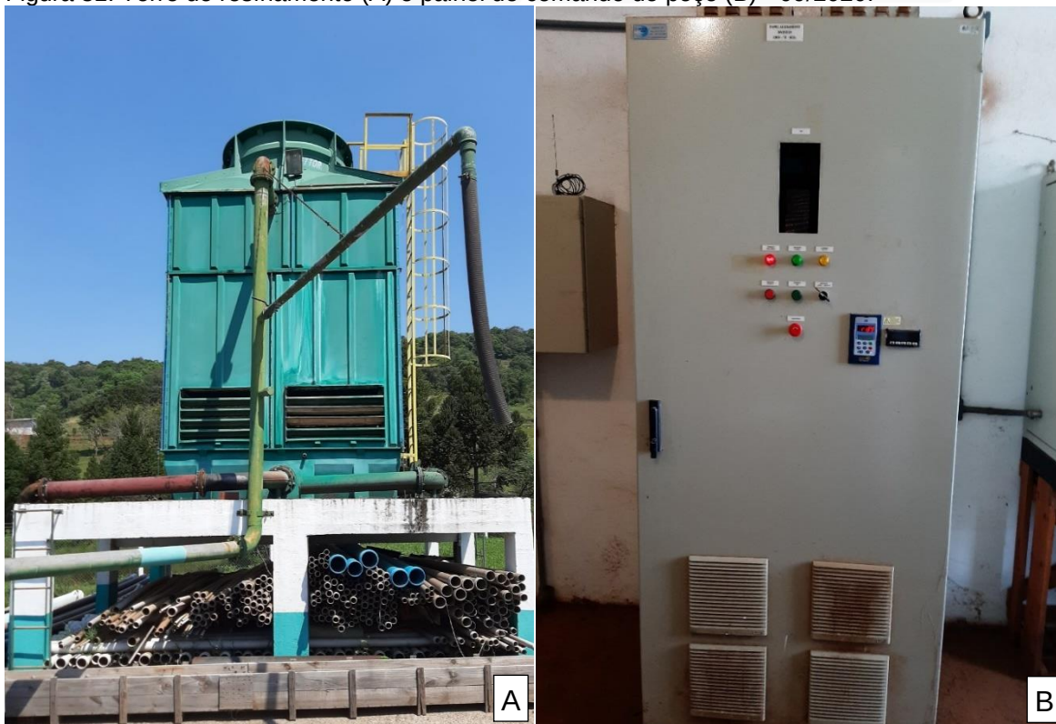
Figura 31: Torre de resfriamento (A) e painel de comando do poço (B) - 09/2020.
