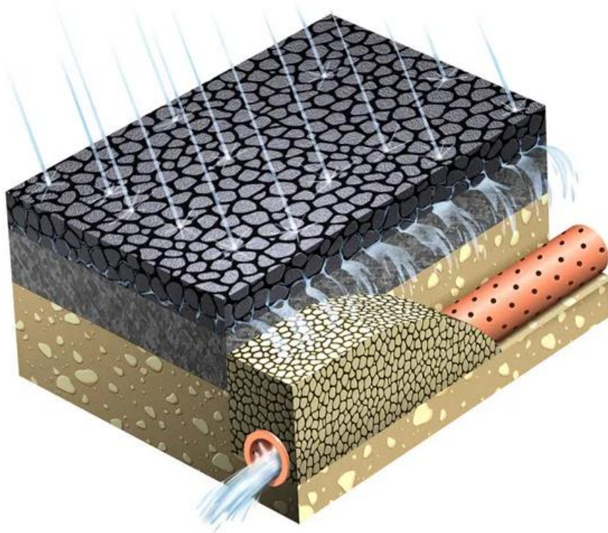
Figura 198: Exemplo de sistema de asfalto permeável.
