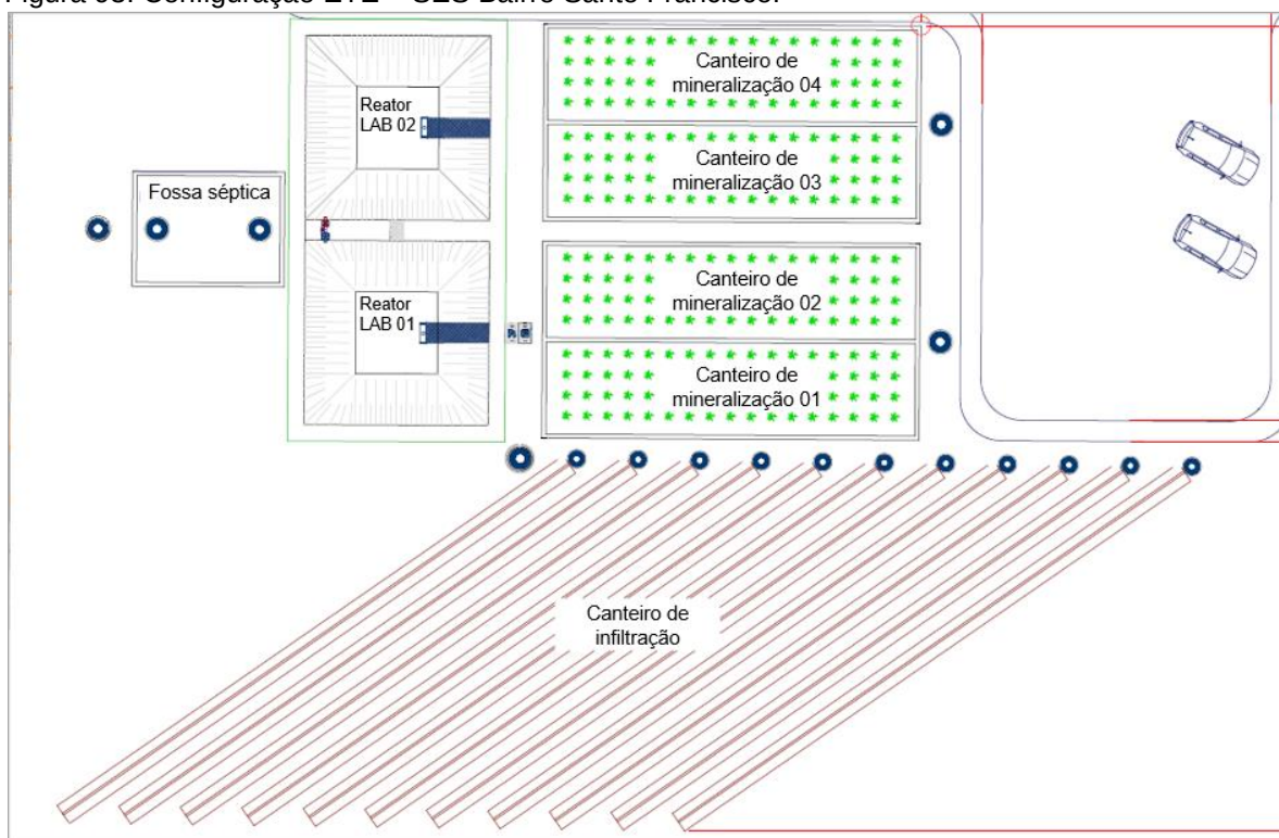
Figura 93: Configuração ETE – SES Bairro Santo Francisco.
