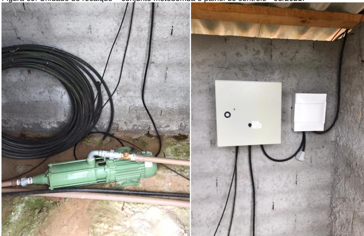
Figura 69: Unidade de recalque – conjunto motobomba e painel de controle - 03/2021.
