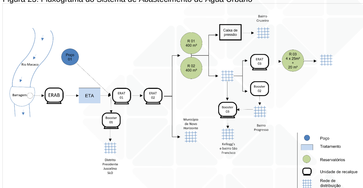
Figura 23: Fluxograma do Sistema de Abastecimento de Água Urbano
