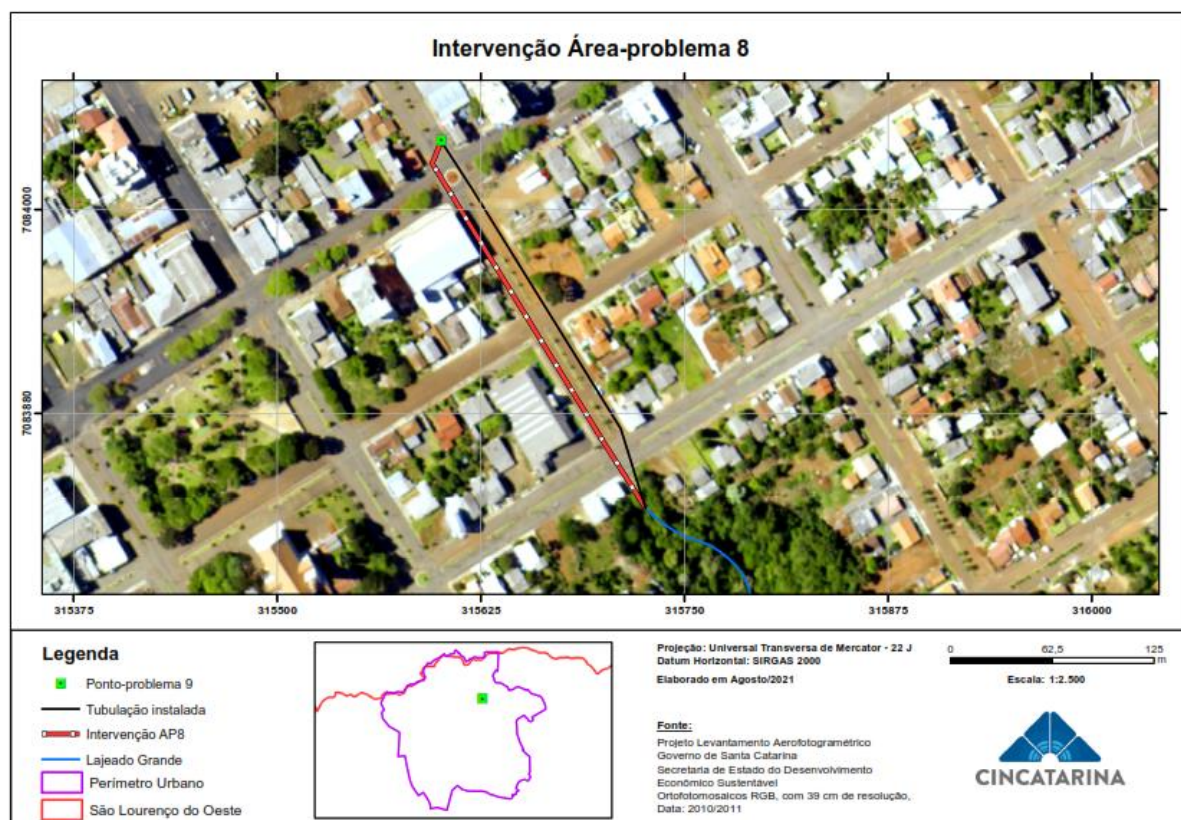
Figura 199: Sugestão de trajeto para o extravasor do Lajeado Grande.
