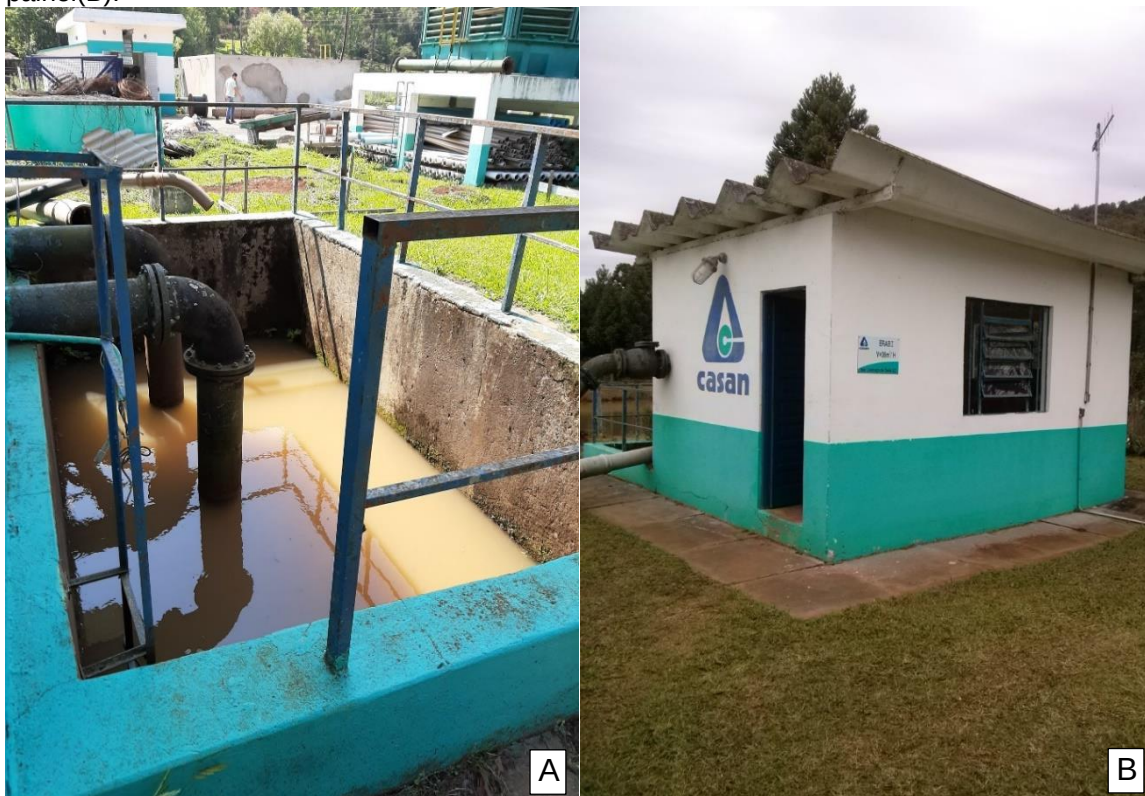
Figura 27: ERAB –Poço de sucção (A) e estrutura civil para proteção do conjunto motobomba e painel(B).
